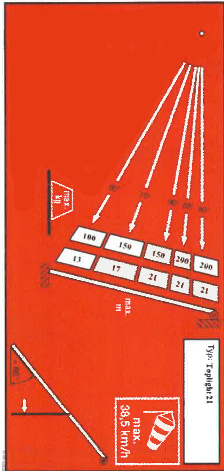
Afb. 4-2 Voorbeeld belastingwijzer Toplight 21/5 meubel
