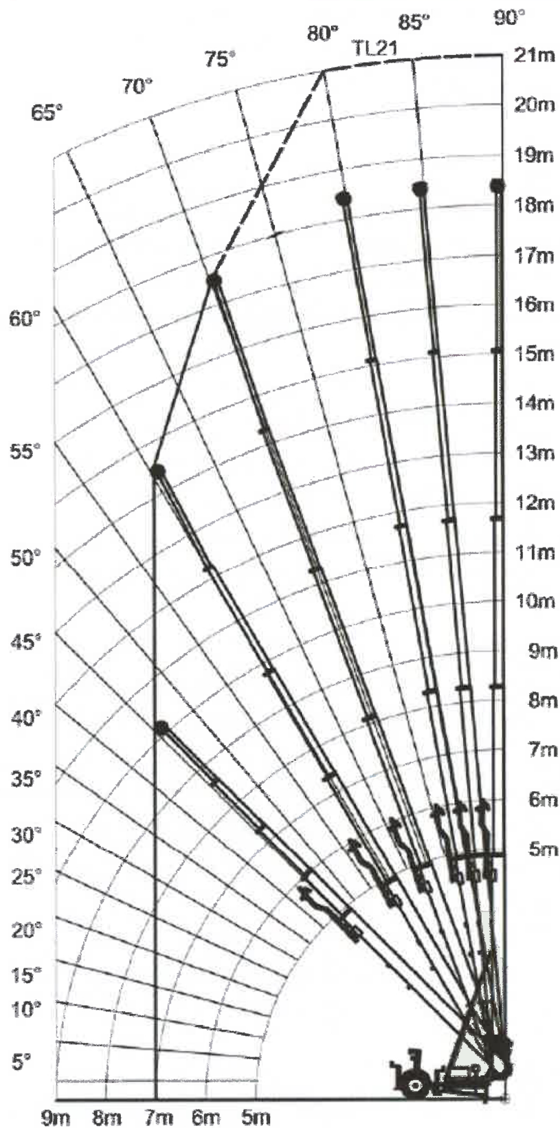
Afb. 4-4 Belastingsgrafiek Toplight 21/5
