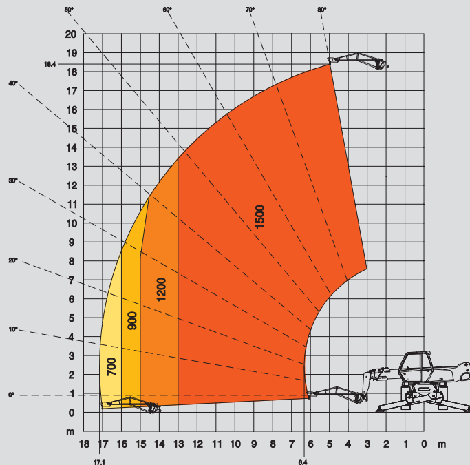
360° ABGESTÜTZT MIT JIB P 1500
